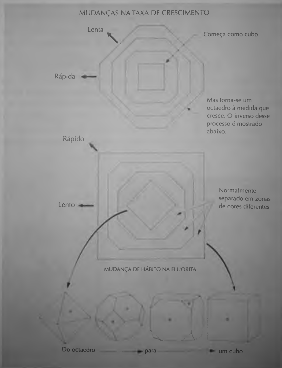
Ilustração 6-36. Um cristal de fluorita.
