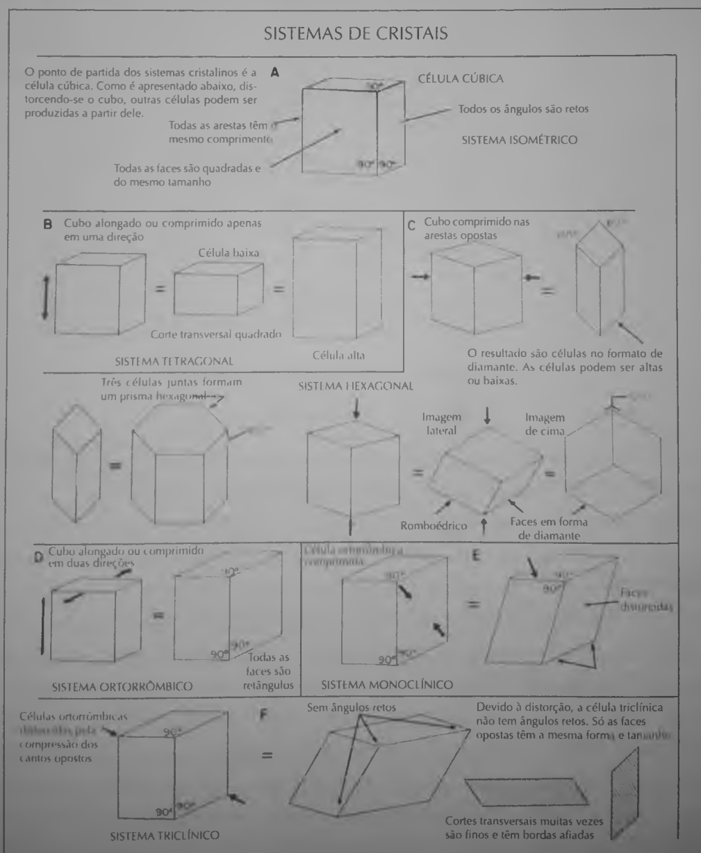
Ilustração 6-34. Sistemas de cristais.
